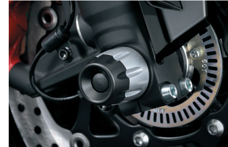
Pádový protektor do hřídele předního kola 54790-48810-000 Snižuje poškození, vyrobený z hliníku a POM (polyacetal).
