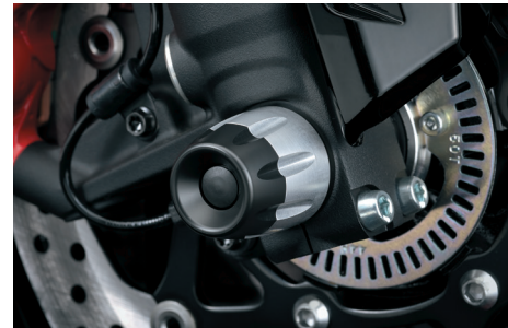
Elsőtengely-protector 54790-48810-000 Hozzájárul a sérülések csökkentéséhez, alumíniumból és poliacetálból (POM) készült.
